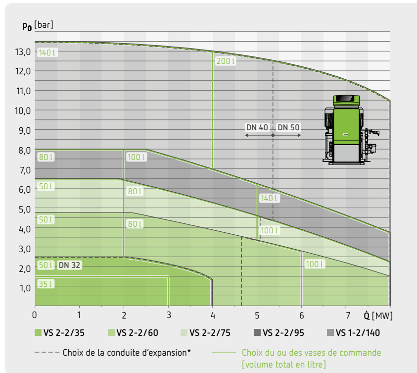
Variomat avec deux pompes
