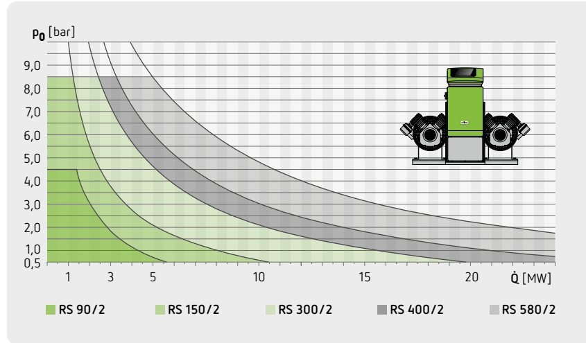
Unité de commande Reflexomat avec deux compresseurs
