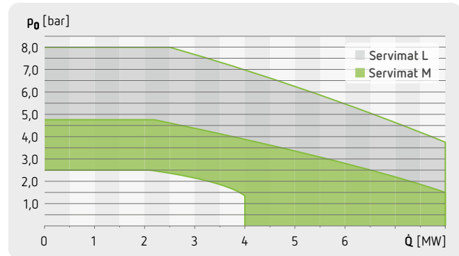
Servimat – Puissance thermique totale de l'installation de production de chaleur Q [MW] en fonction de p_0
